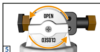
5 Ruotare lentamente la manopola su OPEN
